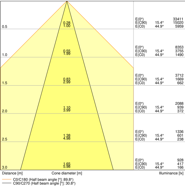
TRUSYS FLEX P 50W 840 VN CL WT EM
