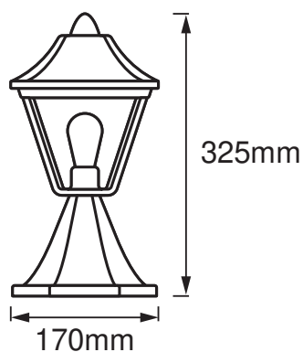
ENDURA CLASSIC TRAD 33CM ALU E27GD
