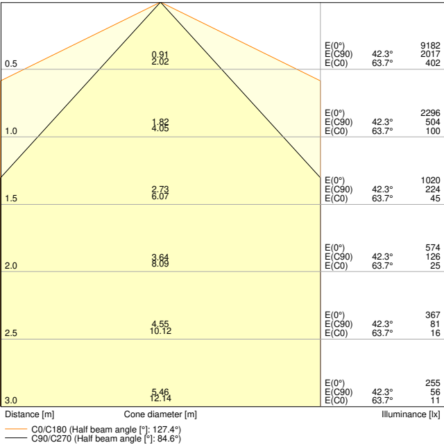
TRUSYS FLEX P 35W 865 W CL WT EM
