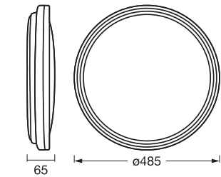
ORBIS HELMAN 485MM 36W 830 WT SI
