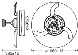
CEILING FAN RETRACTABLE 1070 66W WT
