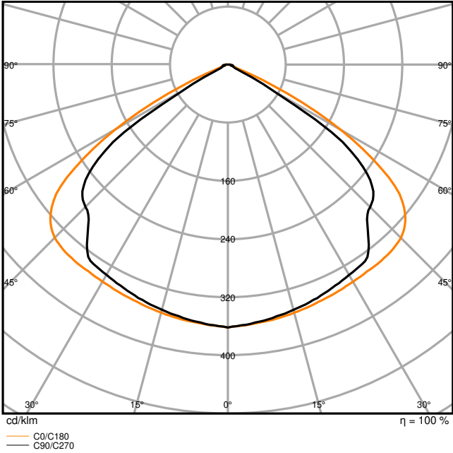
LB FLEX 1500 DALI P 105W 840 VW
