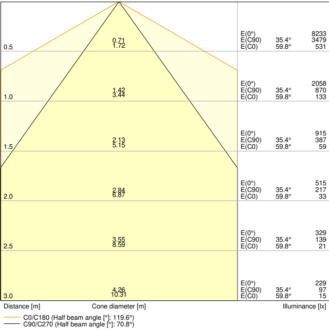
TRUSYS FLEX P 35W 865 DS CL WT EM
