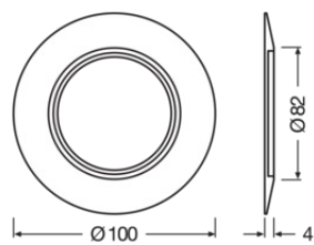
SP RING D100
