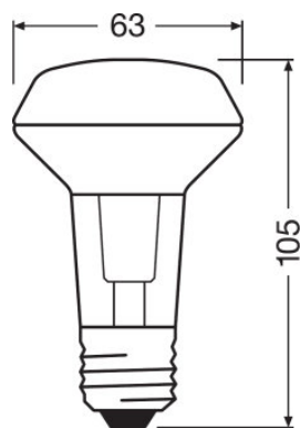
P R63 60 36° 5.9 W/2700K E27
