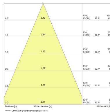
P R63 60 36° 5.9 W/2700K E27
