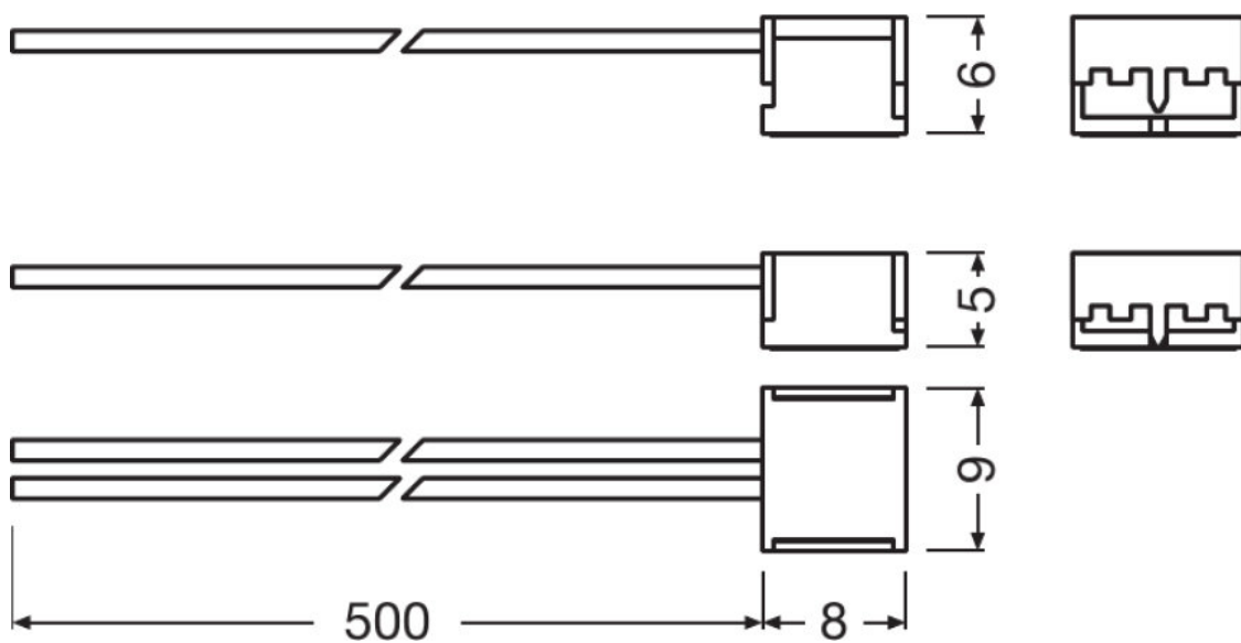
FX -SC08-G2-C2PF-IP54-0500
