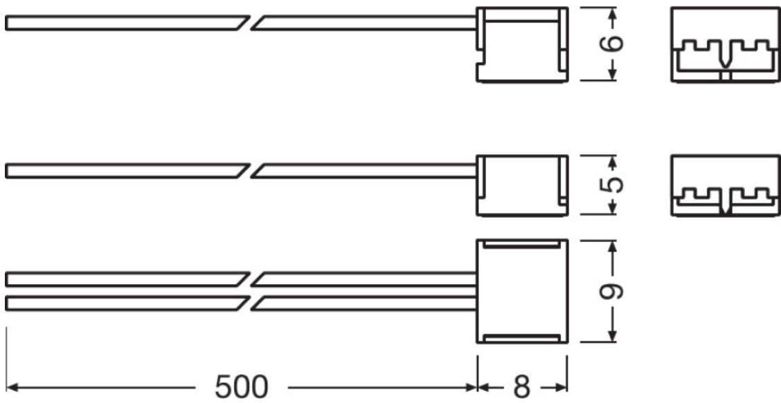
FX -SC08-G2-C2PF-IP54-0500
