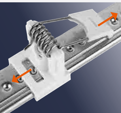
Resortes ajustables para adaptarse al recorte del techo.
